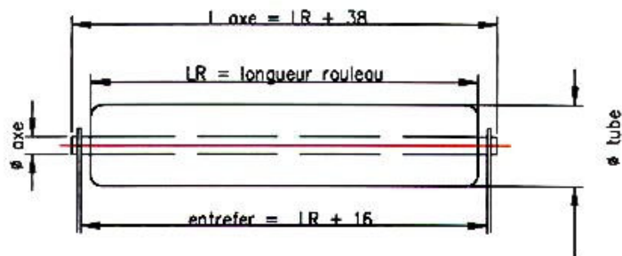
roulement de manutention
