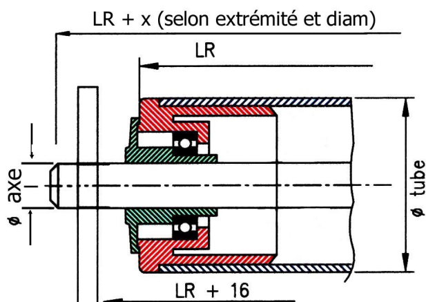
roulement de précision
