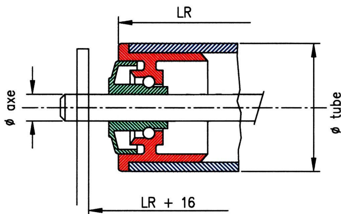
roulement de manutention
